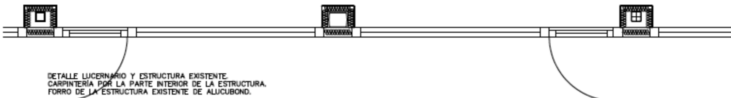
④ L4 LUCERNARIO CON HOJAS FIJAS Y VENTANAS MOTORIZADAS ① UD. VIDRIO EXTERIOR DE 6mm, CONTROL SOLAR BAJO EMISIVO. CÁMARA DE AIRE DE 14mm CON ARGÓN Y VIDRIO INTERIOR DE 5mm, BAJO EMISIVO.
